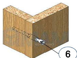
Евровинт 7 x 50
